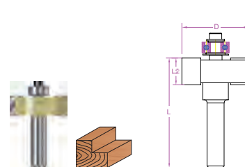
Falzfräser mit Kugellager T-Slotting Bit with Ball Bearing
