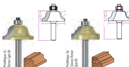
Profilfräser A/B mit Kugellager Roman Ogee Bit/Classical Roman Ogee Bit with Ball Bearing
