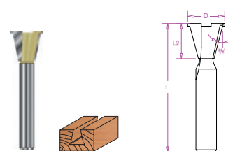
Grat-/Zinkenfräser mit Vorritzer Dovetail Bit with Pre-Cutter
