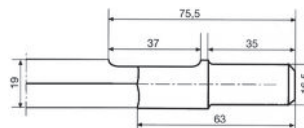
Schaft/Shank 19 mm 6-kant/Hex. Bosch große Keilwelle/Spline
